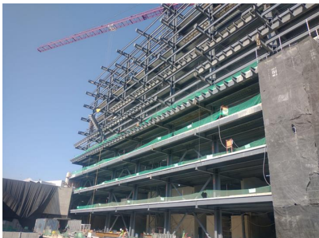
Colocación de acero para fachadas.
