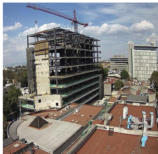
Colocación de acero
